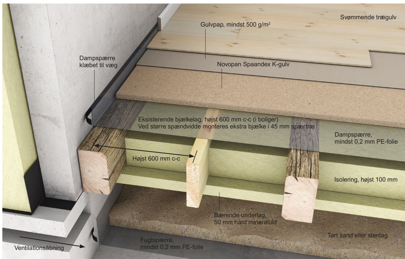
Figur 1 Novopan Spaandex K-gulv lagt på et ældre krybekælderdek og afsluttet med et svømmende trægulv.
